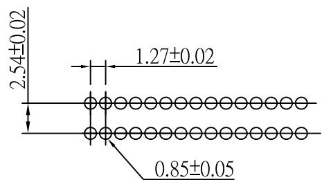
P.C.Board Layout
