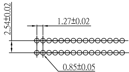
P.C.Board Layout
