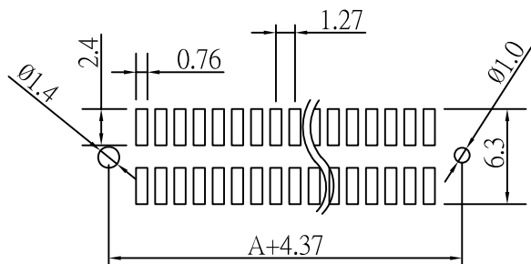
P.C.Board Layout
