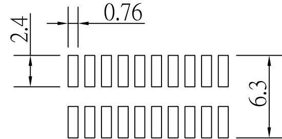
P.C.Board Layout
