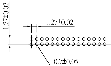
P.C.Board Layout
