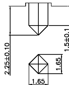
DETAIL: K
