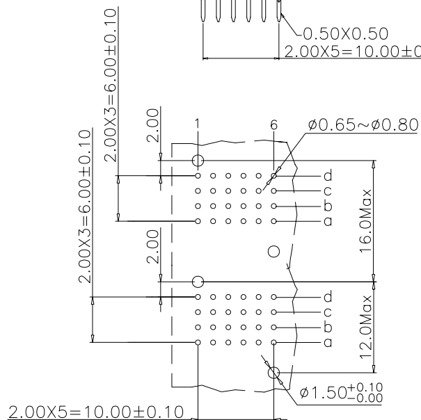
P.C.Board Layout
