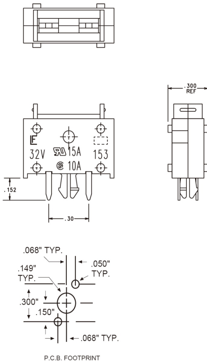
P.C.B. FOOTPRINT
