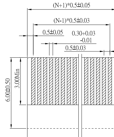
APPLI CABLE FPC
