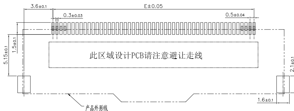
适用线路板 RECOMMENDED PCB LAYOUT
