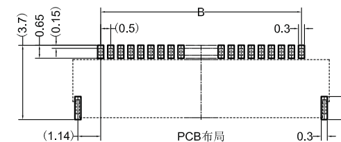
PCB布局
