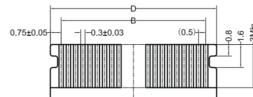
建议排线尺寸 / 厚度0.30±0.03
