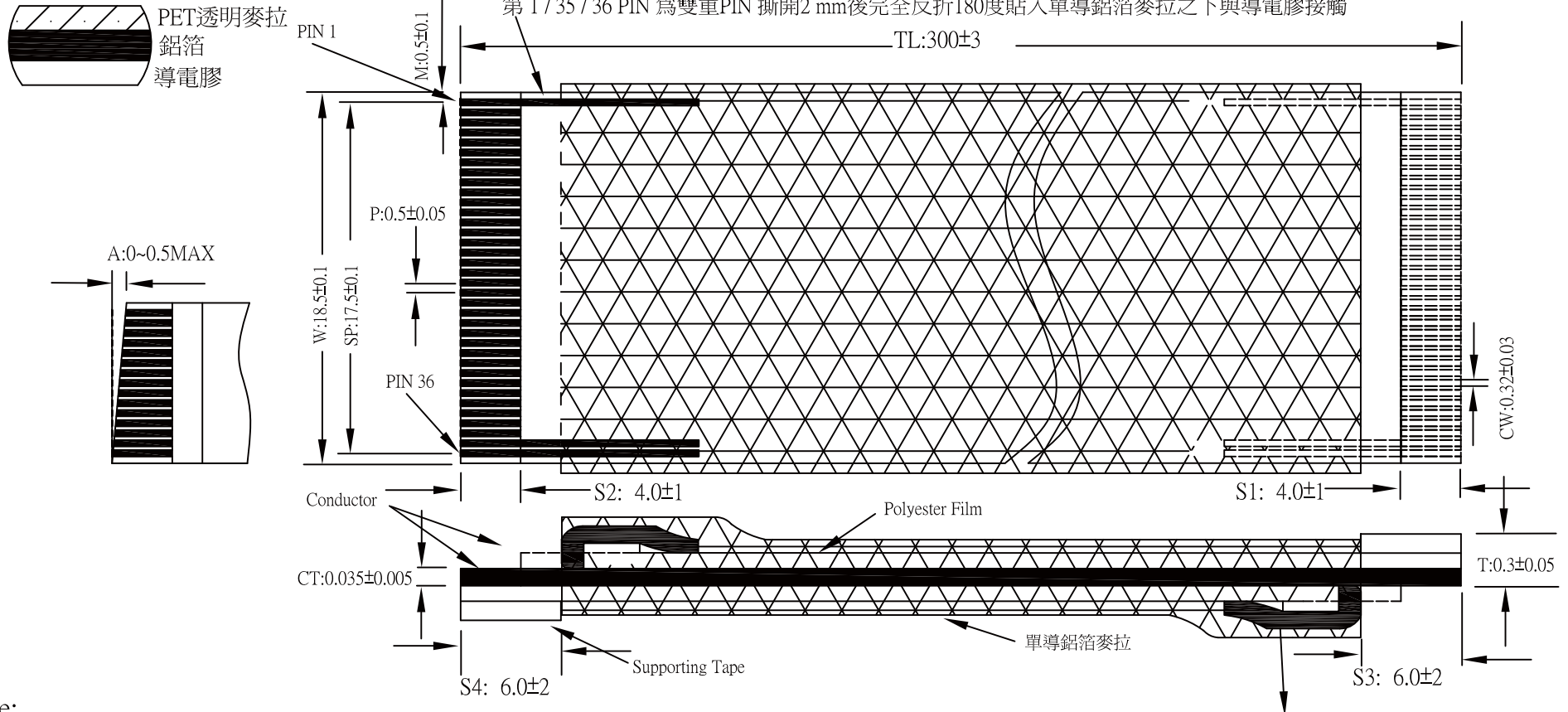
單導鋁箔麥拉結構表示圖
