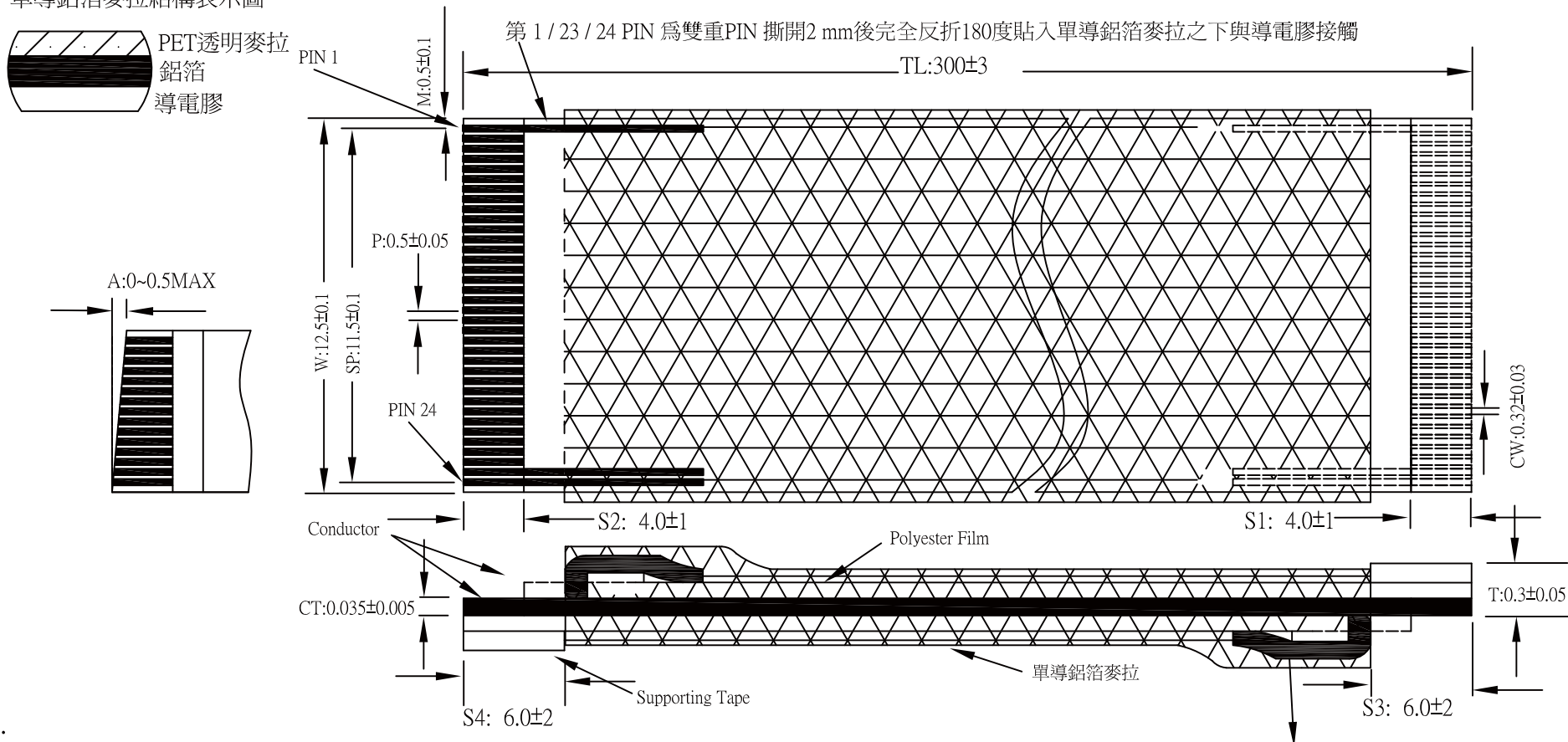
單導鋁箔麥拉結構表示圖
