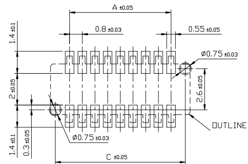
PCB. PATTERN (REF)
