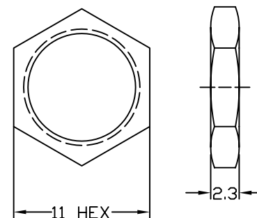
( NUT )
