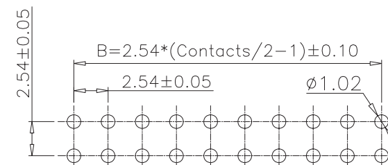
P.C.B. LAYOUT
