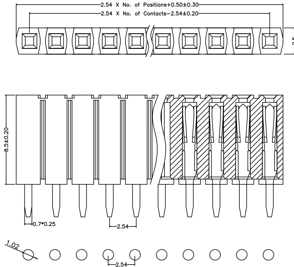
P.C.B LAYOUT
