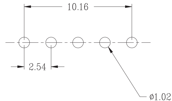
P.C.B. Layout
