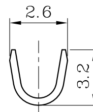
SEC. A-A
