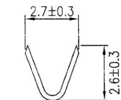
A-A SECTION
