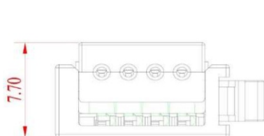
打开状态
