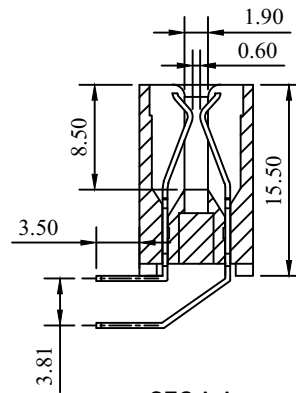
SEC A-A
