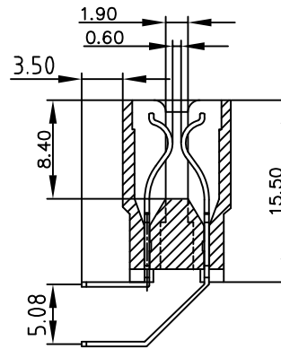
SEC: A-A
