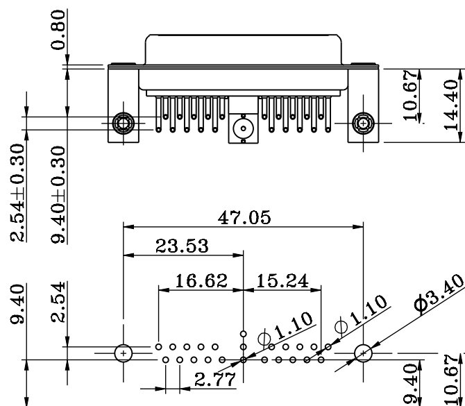
P.C.B. LAYOUT
