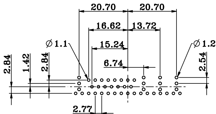
P.C.B LAYOUT
