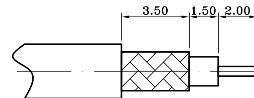
CABLE STRIP
