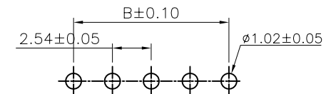
P.C.B. Layout
