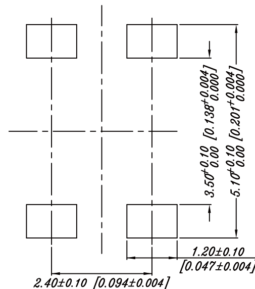
P.C.B. LAYOUT
