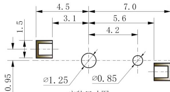
安装尺寸图
