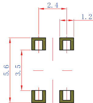
安装尺寸图
