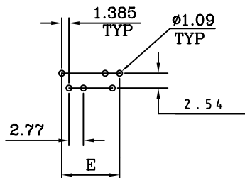
RECOMMEND P.C.B LAYOUT
