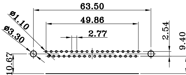
PCB LAYUOT
