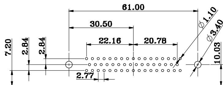
P.C.B LAYOUT
