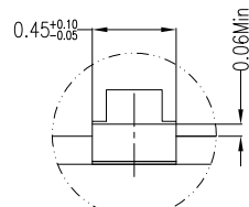
Detail: C Scale 10:1
