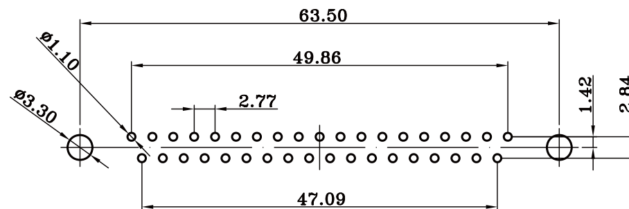
P.C.B LAYOUT
