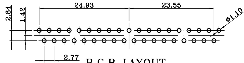
P.C.B LAYOUT
