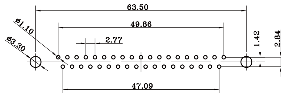
P.C.B LAYOUT
