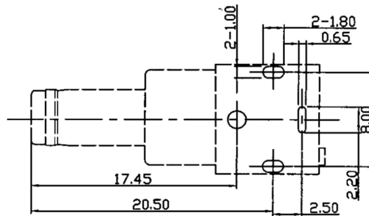
P.C.B Layout/View
