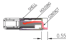
SEC : A--A (2:1)
