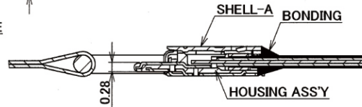
断面図 X-X スケール 10:1
