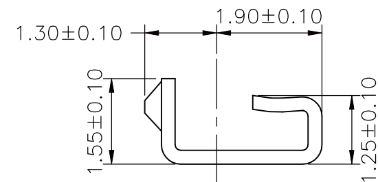
SEC:D-D
