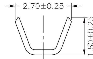
SEC:A-A
