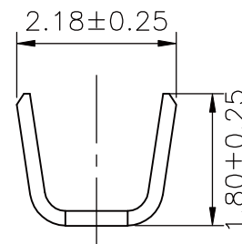
SEC:B-B
