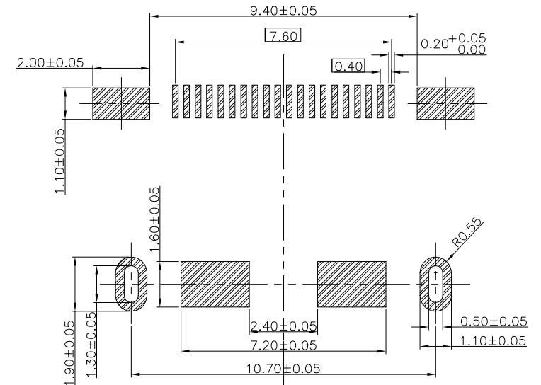
P.C.B LAYOUT
