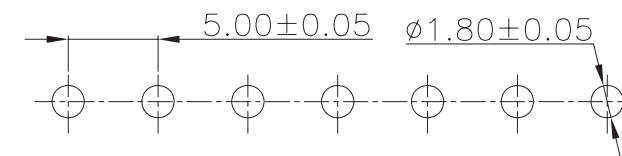
P.C.B Layout
