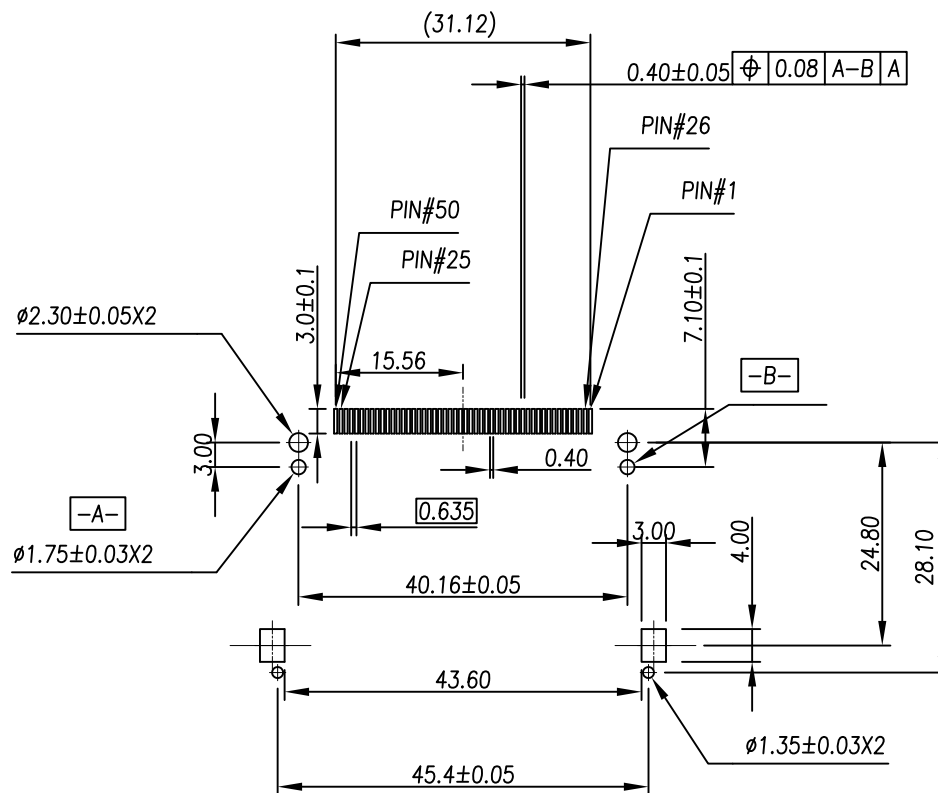
P.C.B Layout
