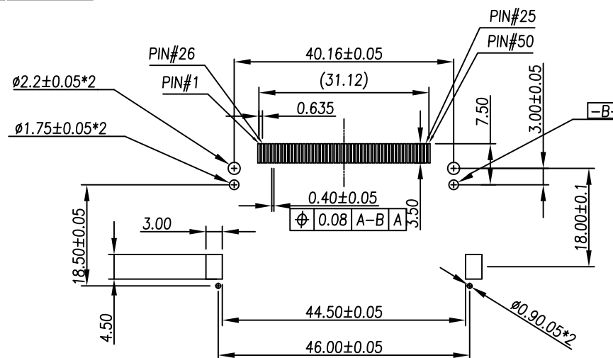
P.C.B Layout
