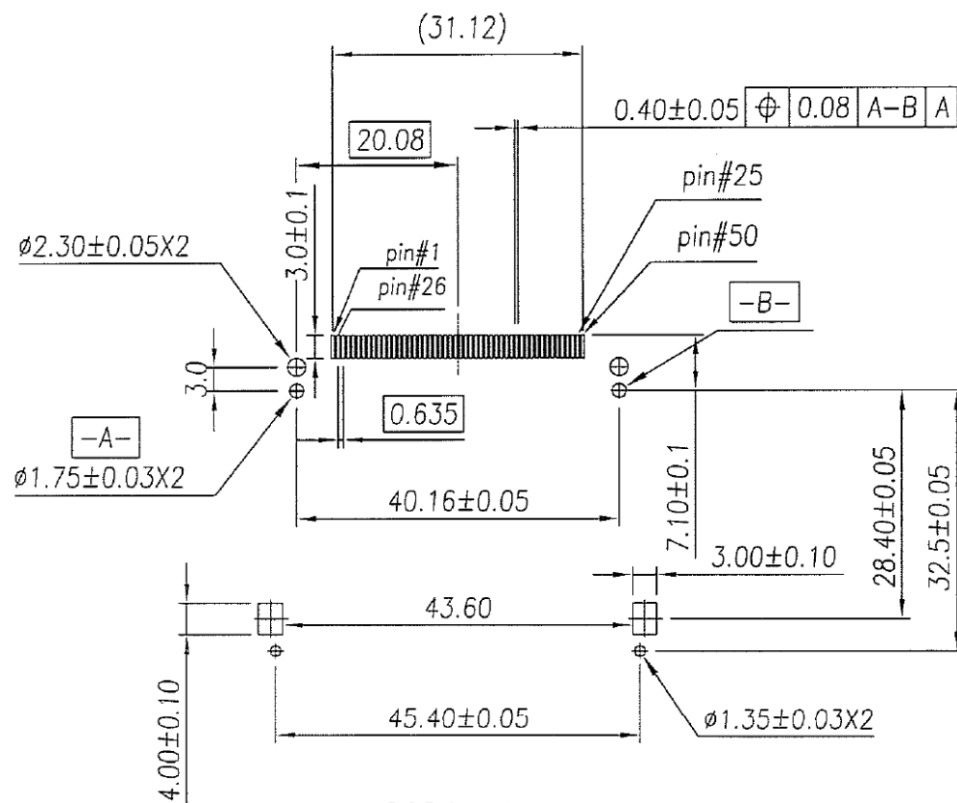
P.C.B Layout
