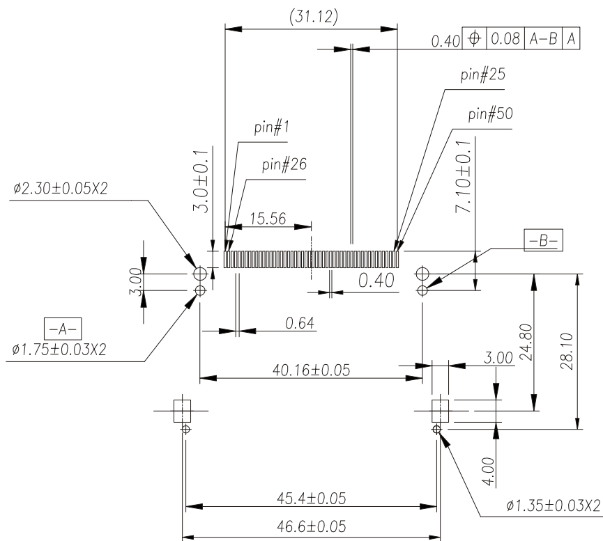
P.C.B Layout
