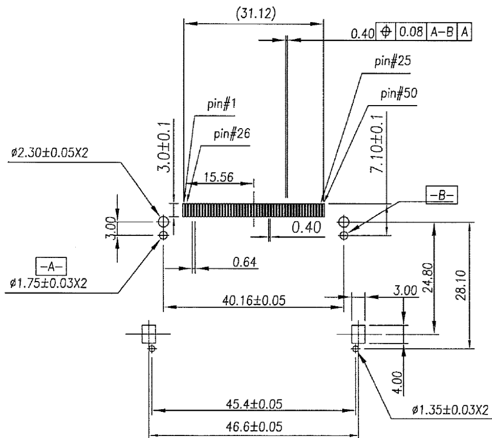
P.C.B Layout
