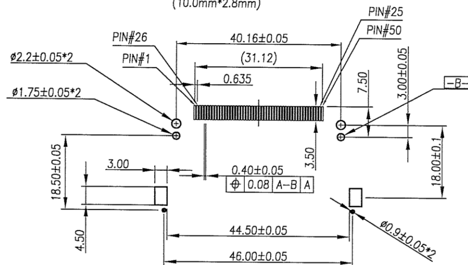
P.C.B Layout
