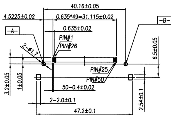
P.C.B Layout
